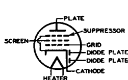
DUPLEX-DIODE PENTODE
