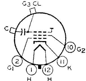
12N ULTOR = G_3 + CL
