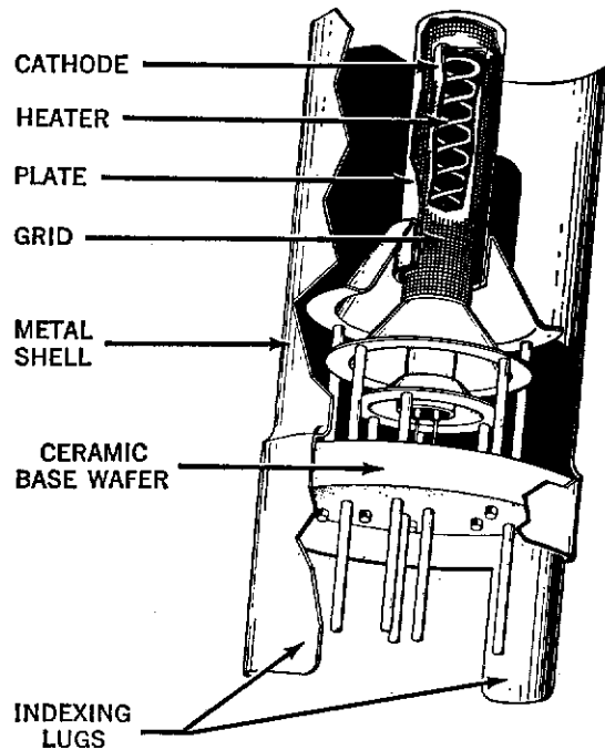
NUVISTOR TRIODE
