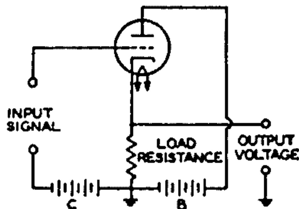
Fig. 51—Cathode-follower circuit.
