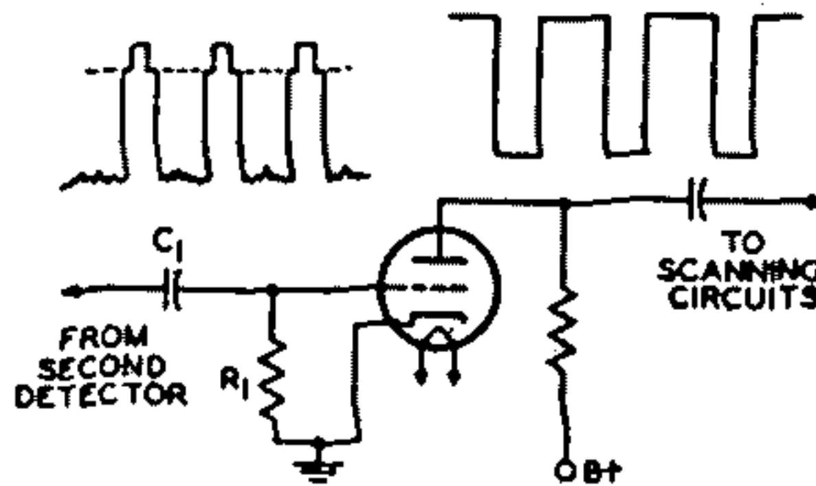
Fig. 80—Sync-separator circuit.
