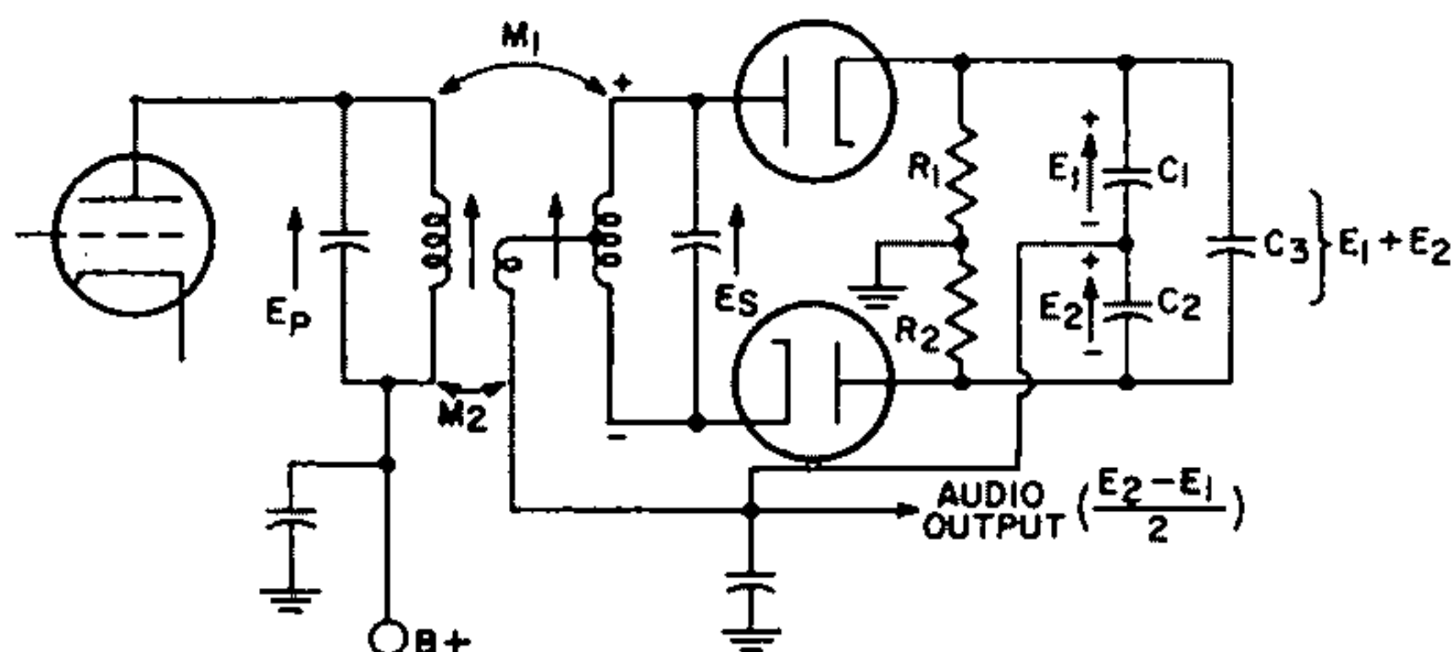
Fig. 33—Radio-detector circuit.
