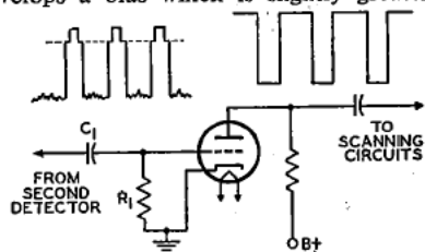
Fig. 80—Sync-separator circuit.
