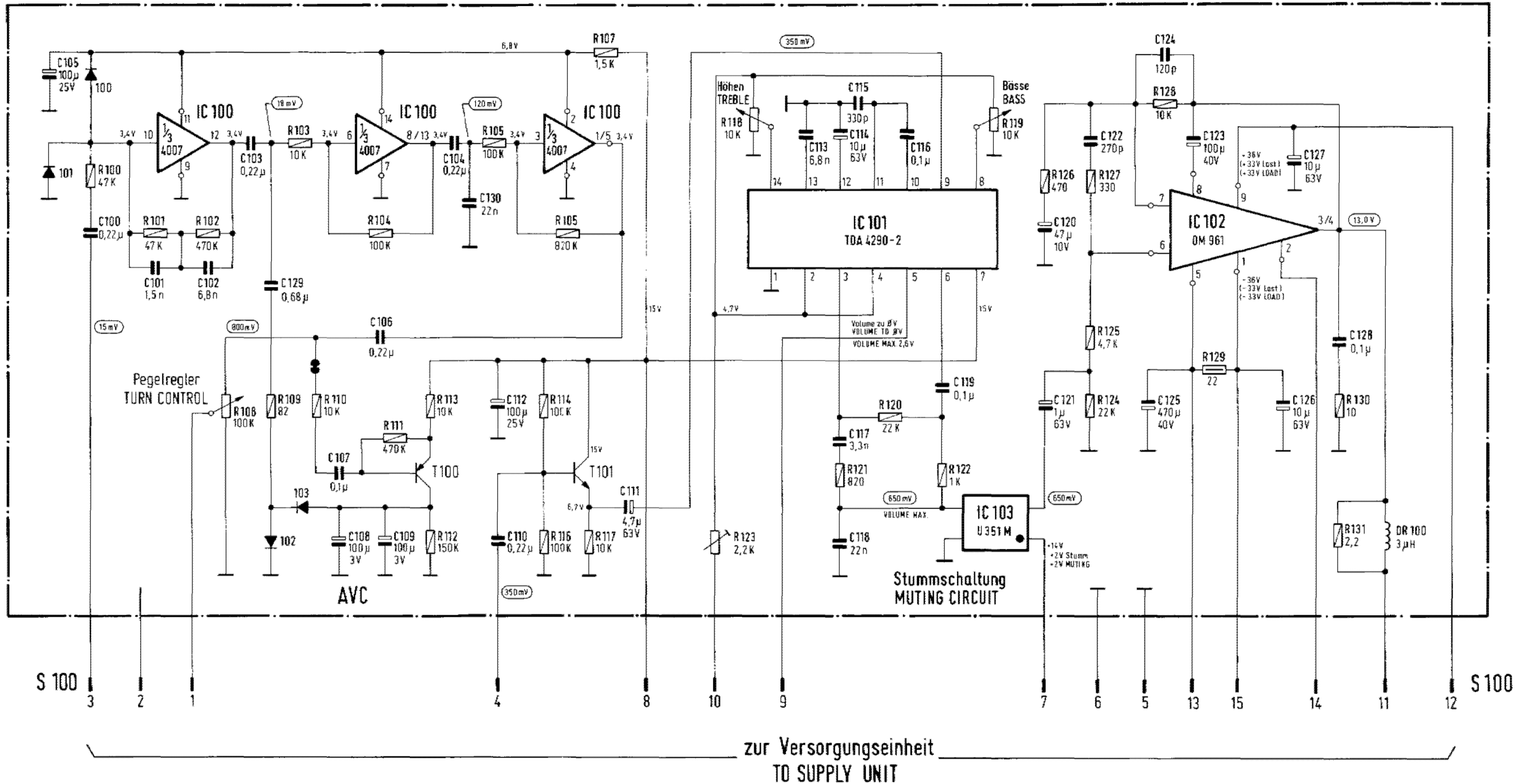
Schaltbild Verstärker WIRING DIAGRAM AMPLIFIER
