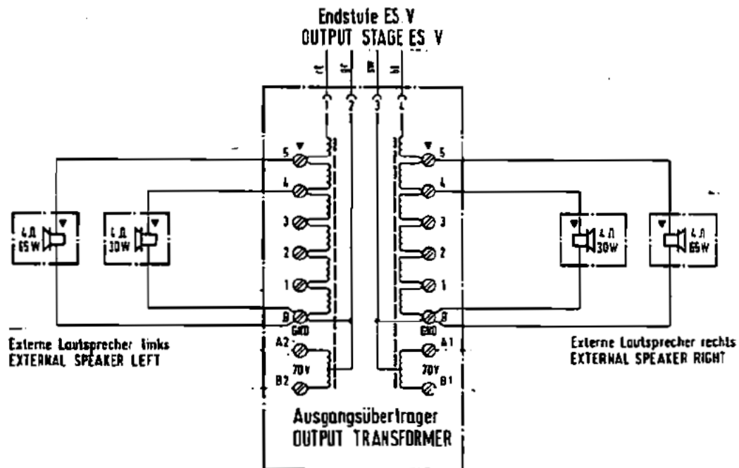
Anschlussschema für Ausgangsübertrager CONNECTION DIAGRAM FOR OUTPUT TRANSFORMER
