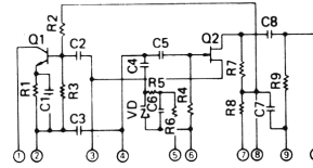
IC-5, UHIC005
