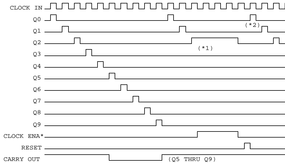
CD4017B
