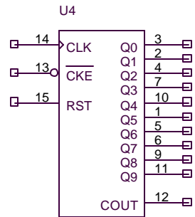
CD4017B
